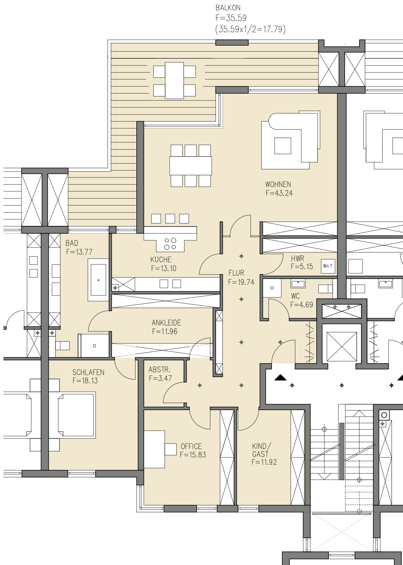
Wohnung 10 – 178,79 m2 mit 5 ZKB
